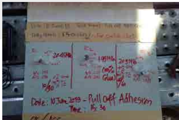
Làm sạch và sơn Ceilcote FGD (Flake Lining) Nhà máy lọc hóa dầu Nghi Sơn
