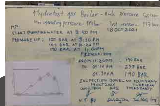
Thử áp lò hơi Unit 1 Nhà máy Nhiệt điện Mông Dương 2
