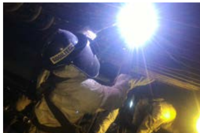
Sửa chữa ống vách lò hơi - Nhà máy Nhiệt điện Mông Dương 2
